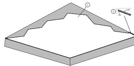
M572 Montageanvisning (M572) for Clipso SO Classic, loftmontage med PCC profiler.
