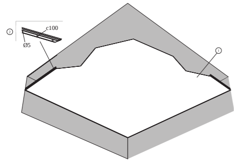
M569 Montageanvisning (M569) for Clipso SO Classic, loftmontage med PCW profiler.
